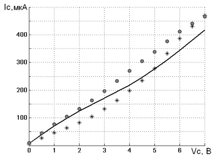
Рис. 5. ВАХ беззатворной гетероструктуры с КТ. Сплошная линия – эксперимент, точки – результаты расчетов для концентрации КТ 3 \cdot 10^{10} см ^{-2} .
