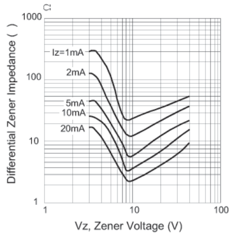
Fig. 4 Typical Zener Impedance vs. Zener Voltage
